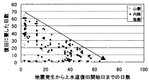
図3 上水道の復旧開始時期と復旧に要した日数
