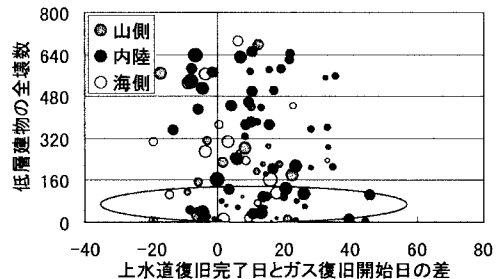
図5 上水道とガスの復旧活動における相互影響
