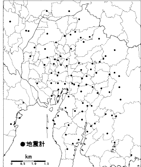
図-1 名古屋地域の地震計配置図
