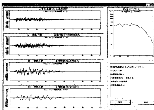
図8 加速度波形および応答スペクトル(皿種地盤)
