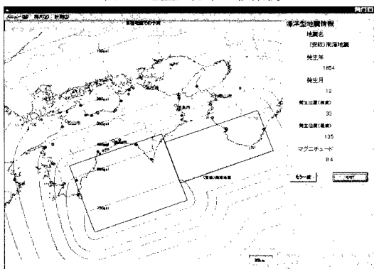
圖 6 最大加速度分布圖(Ⅲ種地盤)
