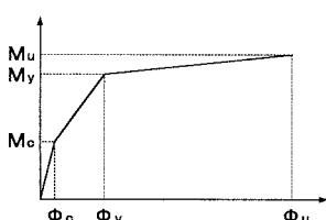
図-2 M- \phi 関係
