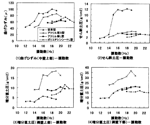
図3 共振曲線
