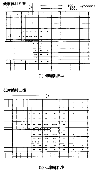
図4 地盤の \sigma_x
