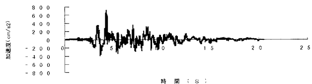
合成加速度波形 (GL-83m)
