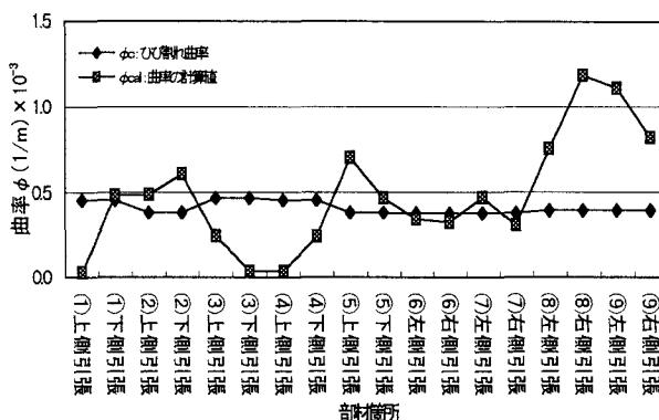
図-5 時刻歴逐次応答解析結果
