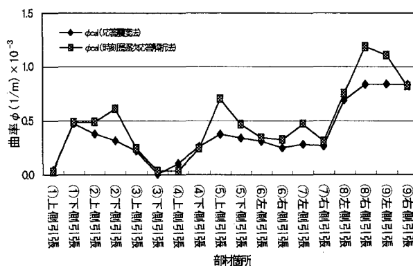
図-6 応答震度法による解析結果
