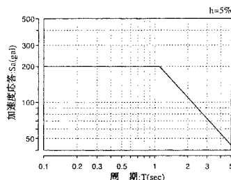
図3 L1標準加速度 応答スペクトル
