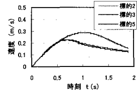
(b) 解析による速度の時刻歴
