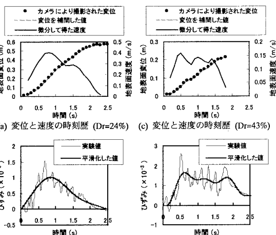
(b) 杭のひずみの時刻歴 (Dr=24%) (d) 杭のひずみの時刻歴 (Dr=43%)
