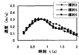
図 5 実験による速度の時刻
