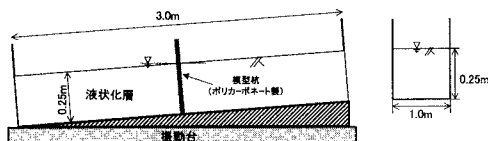
図 1 杭―地盤模型の概要
