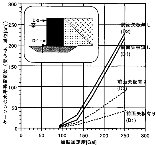
図一2 加振加速度とケーソンの残留変位
