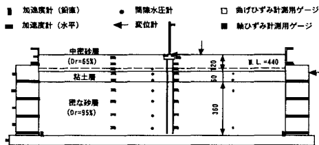
図1 遠心振動実験模型（配管基礎モデル）
