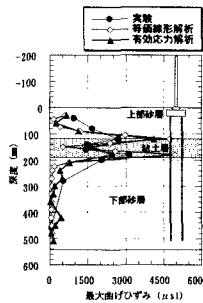
図5 杭の曲げひずみ最大値分布
