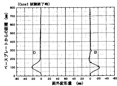
図-6 局部座屈膨らみ形状
