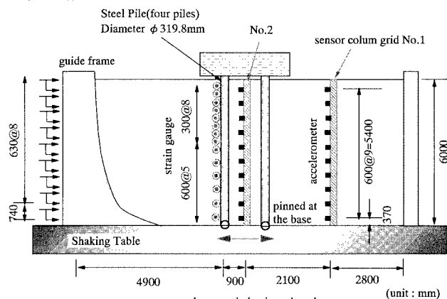
図1 実験概要
