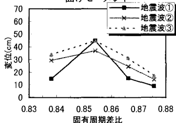
a) 隣接径間を考慮しない場合
