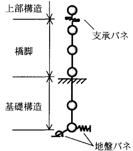
図2 解析モデル（詳細）
