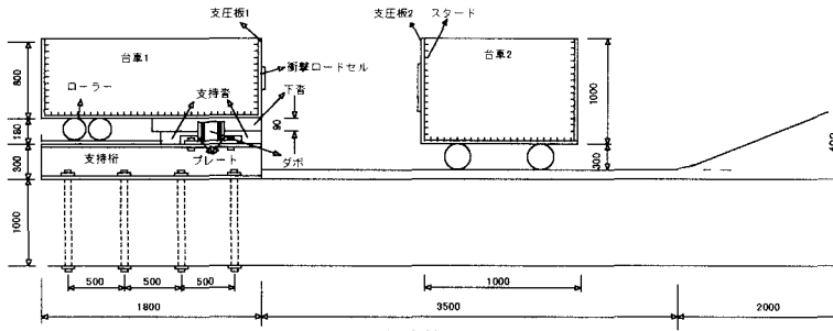
図-1 実験装置
