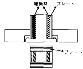
図-2 緩衝材とプレートの挿入
