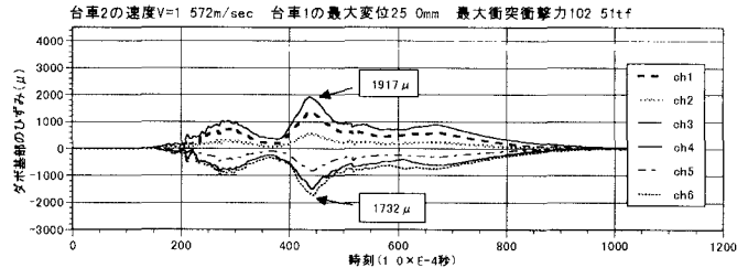
図-7 緩衝材同じ向き (a) の場合のひずみ-時刻の関係
