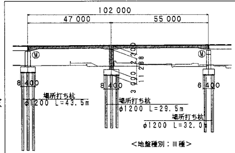
図-1 対象橋梁
