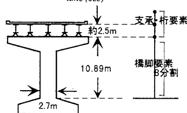
図2 解析モデル
