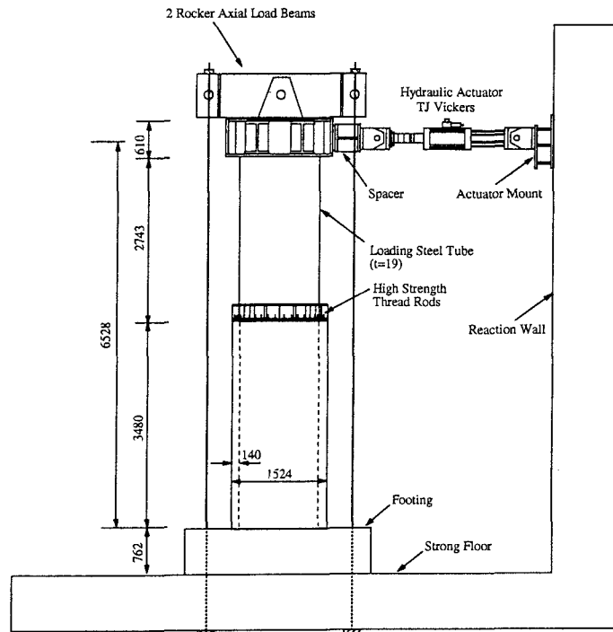
Fig. 1 Test Setup
