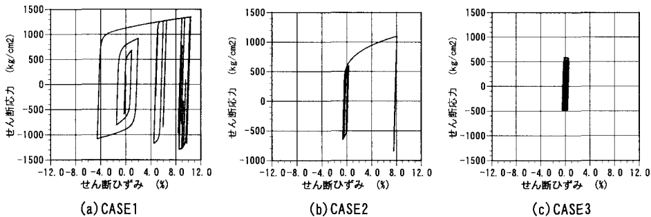
図－6 塑性履歴ループ
