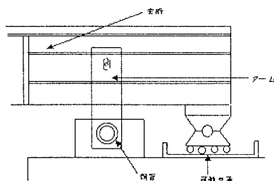
図-1 吸振装置
