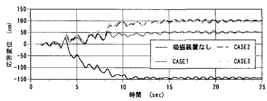
図－5 (b) 可動支承部の橋脚応答変位
