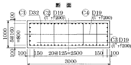
図-1 橋脚モデル（橋脚高4m）
