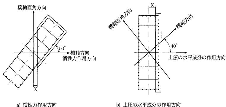
図-2 断面算定方法
