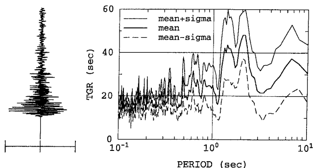
図-1 袖ヶ浦の地表記録の時刻歴と群遅延時間
