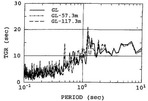
図-3 群遅延時間の標準偏差の比較(袖ヶ浦・地表と地中)
