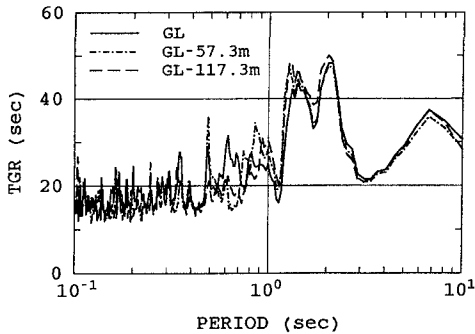
図-2 群遅延時間の平均値の比較(袖ヶ浦・地表と地中)
