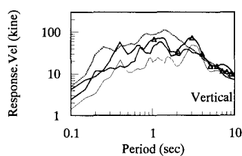
図-7 FEM地表面の各鉛直応答（解析SV-P波入射）
