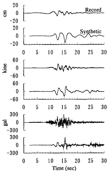
図-4 KBUにおける解析波形と観測波形の比較（EW成分）
