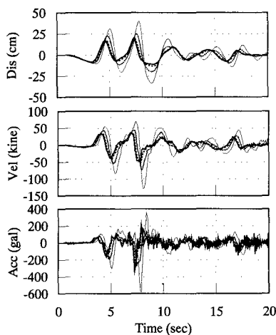
図-3 KBUにおける解析波形と観測波形の比較（NS成分）
