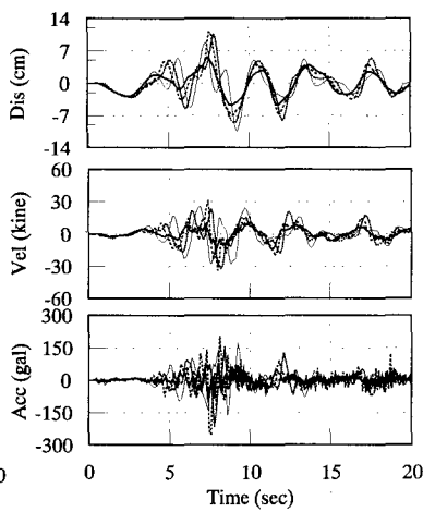
図-4 KBUにおける解析波形と観測波形の比較（EW成分）
