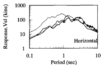
図-6 FEM地表面の各水平応答（解析SV-P波入射）
