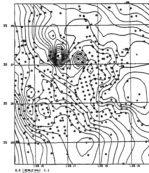
図 3: ブーゲー異常図 (仮定密度 2.45):0.5mgal 間隔
