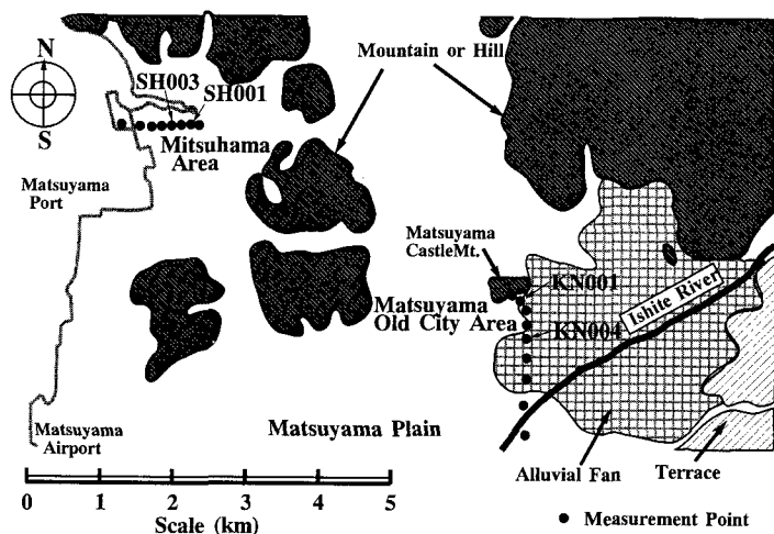
図-1 測定対象地域のある松山市北部の地質と測定点
