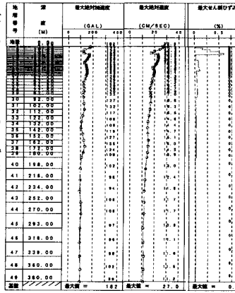
図-6 第二工業港地盤応答
