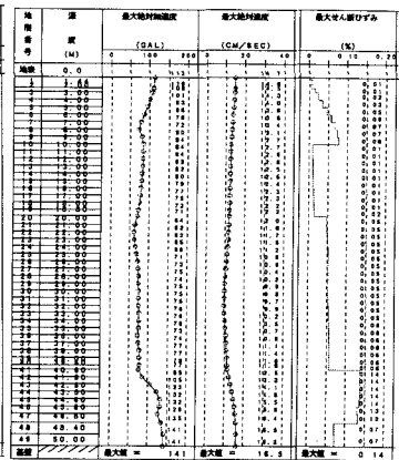
図-7 第一工業港地盤応答
