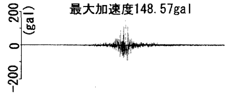
図-5 三陸はるか沖地震地震動
