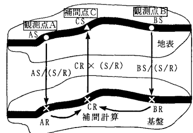
図－1 観測地点間の地震動推定方法
