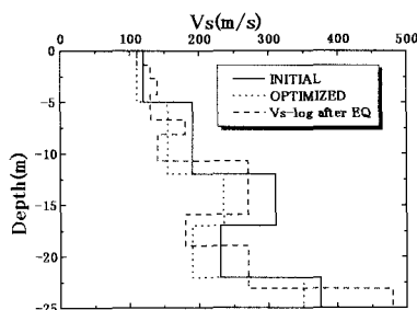
図2 S波速度の同定前後の比較
