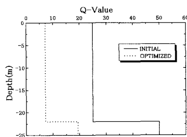
図3 Q値の同定前後の比較
