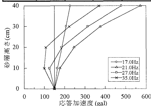
図-5 150gal増加時の高さ10cmと応答加速度の関係
