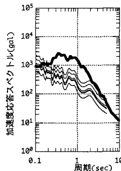
図4 大正関東地震
