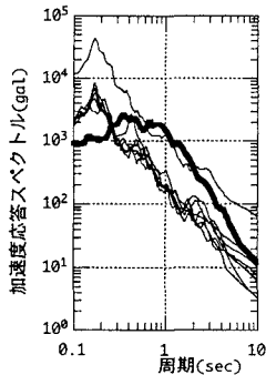
図2 北武断層M7
