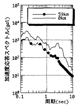
図5 断層深さの影響
