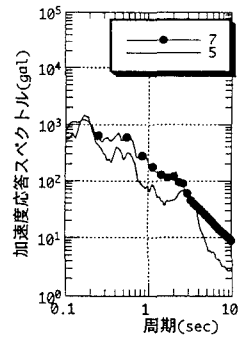
図6 重ね合わせ数の影響
