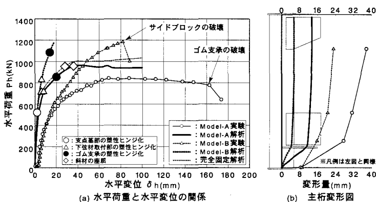
図-5 耐荷力実験およびFEM解析結果
