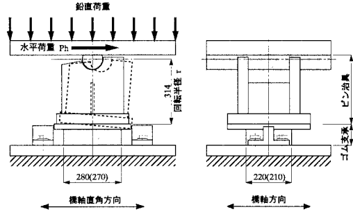
図-1 ゴム支承の耐荷力実験概要図
