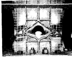
Photo.2 座屈状態例 (Type-SD)
