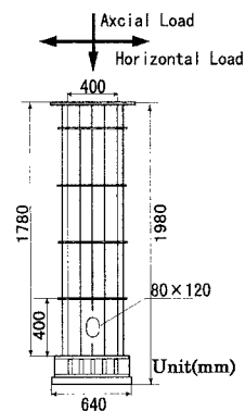
Fig.1 実験供試体
