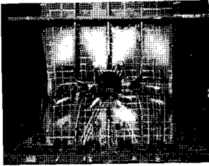
Photo.1 座屈状態例 (Type-H)
