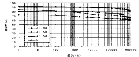
図-7 たわみからの合成度
