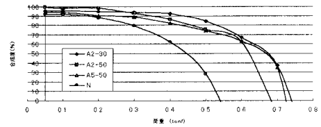
図-3 ひずみからの合成度
