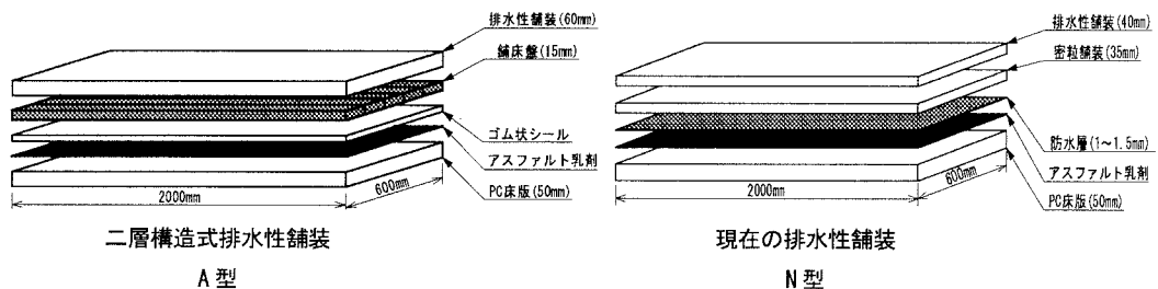
図-2 試験体の構成
