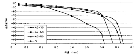
図-4 たわみからの合成度
