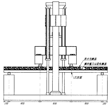
図-1 試験体と載荷状態
