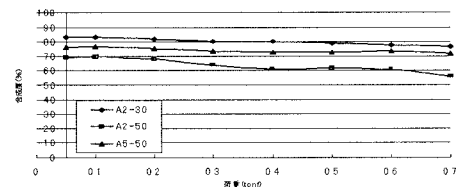
図-5 ずれからの合成度
