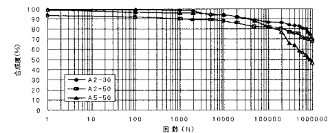
図-8 ずれからの合成度
