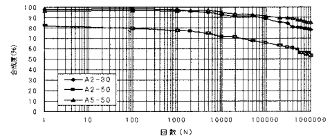
図-6 ひずみからの合成度
