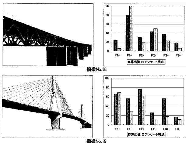
Fig. 3 橋梁形態の写真例及び算出値とアンケート得点によるプロフィール比較図
