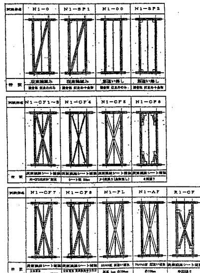
図 2-2 試験体一覧
