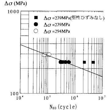
図-4 S-N 線図
