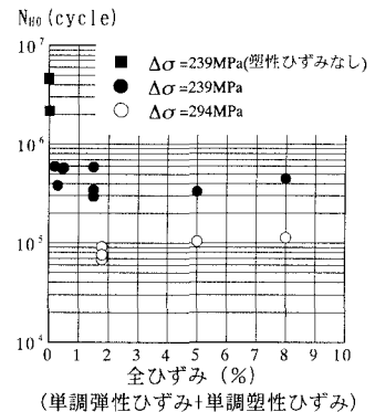
図-3 単調塑性ひずみの影響
