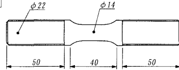
[平行試験片]
