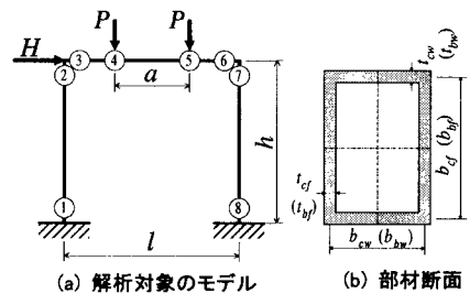
図-1 解析対象の構造物
