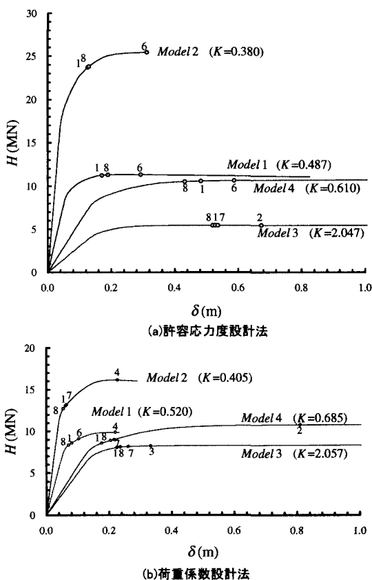
図-2 鋼製ラーメン橋脚の水平耐力と水平変位の関係
