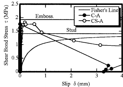
図 2 ずれ挙動(押抜き試験法)
