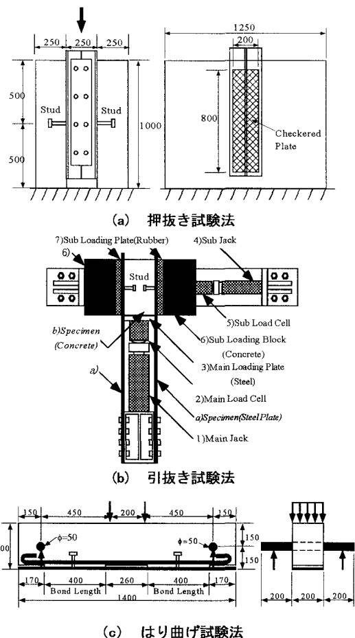
図 1 各種試験法の供試体
