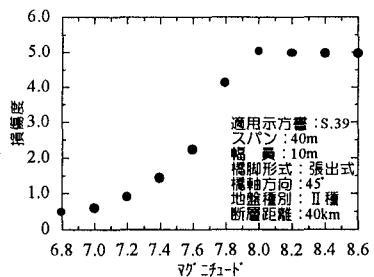
図-5 マグニチュードと損傷度の関係
