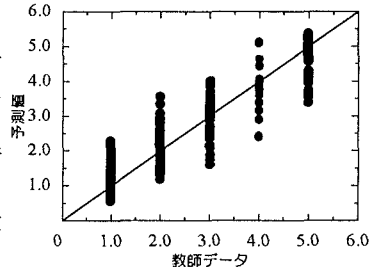
図-4 教師データと予測値の関係
