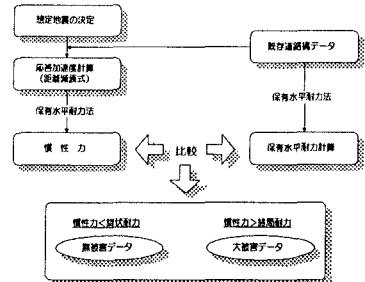
図-3 架空データの作成概要
