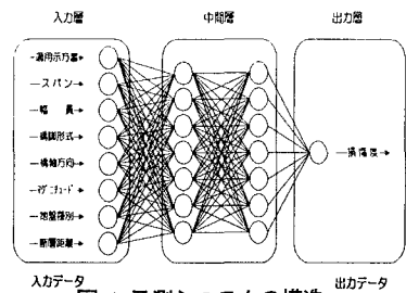
図-1 予測システムの構造
