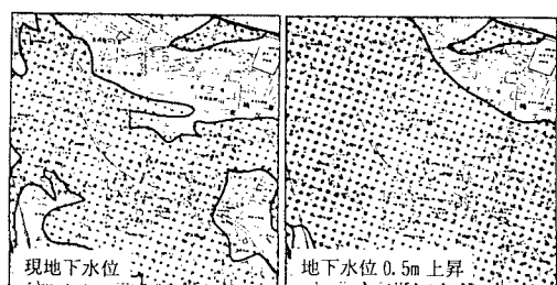
図-5 レベル2地震動下での自然堤防地帯における 現地下水位と地下水位 0.5m 上昇時の予測結果
