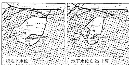
図-6 レベル2地震動下での三角州地帯における 現地下水位と地下水位 0.2m 上昇時の予測結果
