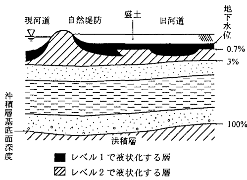
図-2 液状化層の概念図
