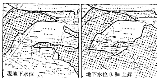
図-4 レベル1地震動下での三角州地帯における 現地下水位と地下水位 0.8m 上昇時の予測結果
