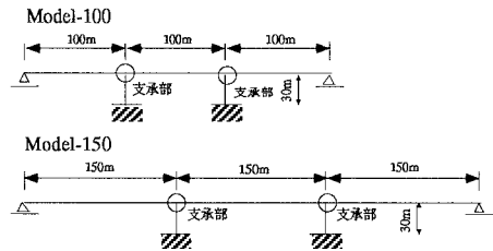
図-1 解析対象モデル
