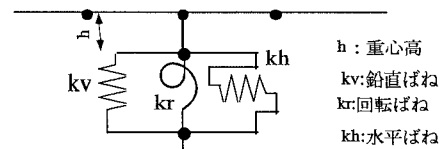
図-2 支承部の解析モデル化
