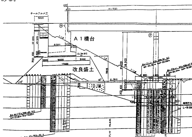
図-1 A1橋台付近地層断面図
