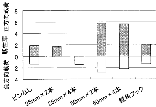
(a)直角フック
