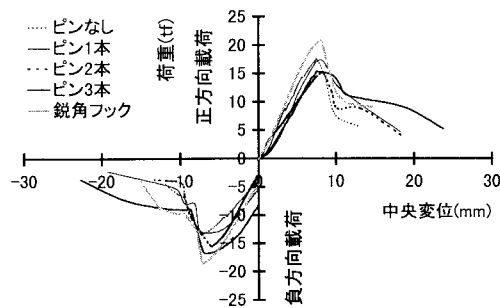
(c)重ね継手 ピン定着長 25mm
