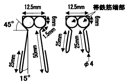
(a)ピン定着長 50mm (b)ピン定着 25mm
