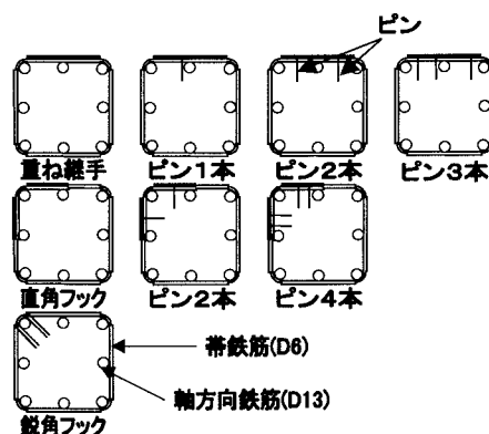
図-2 ピンの本数および設置位置図
