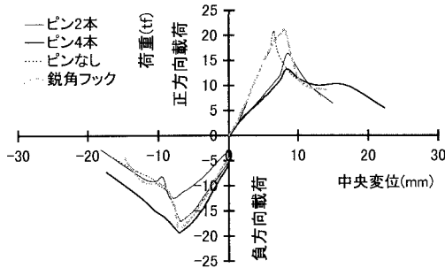
(a)直角フック ピン定着長 25mm
