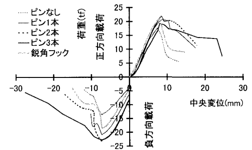
(d)重ね継手 ピン定着長 50mm
