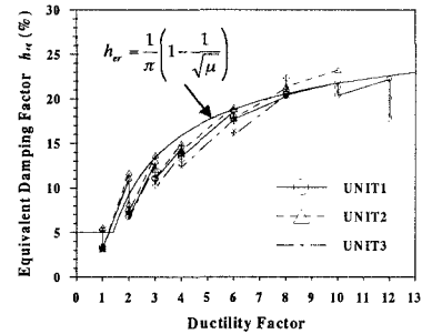
図3 等価粘性減衰定数
