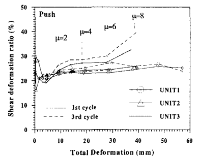
図4 せん断変形分担率
