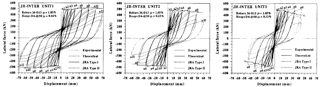
図2 荷重－変形関係
