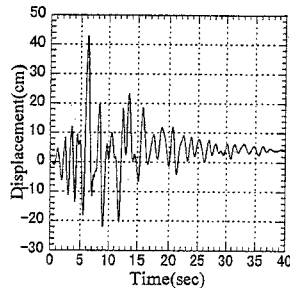
図7 時刻歴応答変位曲線
