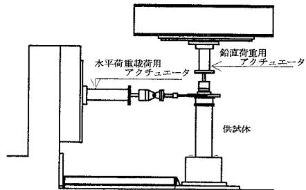
図2 載荷装置図
