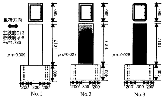
図1 供試体形状
