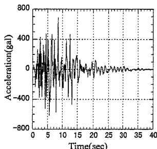
図5 入力加速度波形
