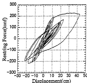
図6 荷重-変位曲線
