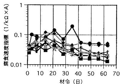
図3 腐食速度指標経時変化
