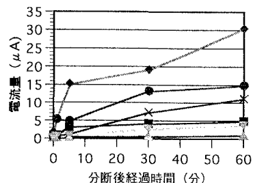
図5 分断後の経過時間と電流量の関係
