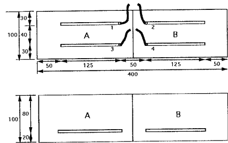
図1 供試体略図
