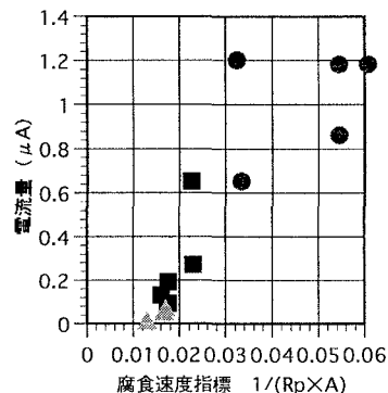
図6 腐食速度指標と電流量の関係
