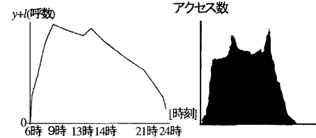
図4: 需要が連続的に発生する場合
