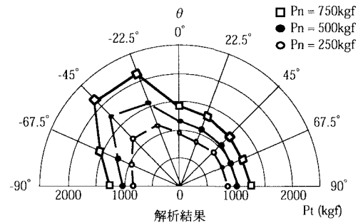
図4 一面せん断試験の結果と解析結果の比較
