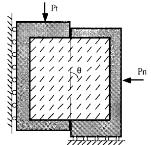
図2 石膏供試体の一面せん断試験
