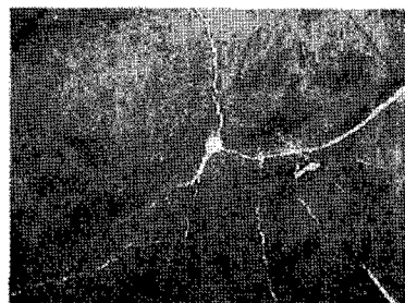
写真2 割裂脈の分布状況(動的注入：DYN2)
