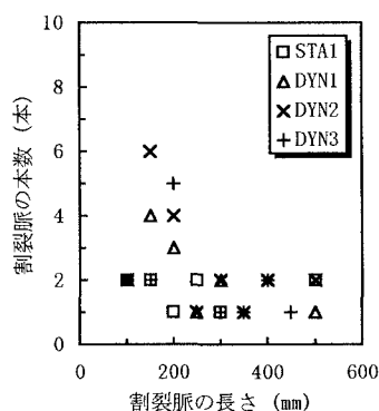
図3 割裂脈の本数と長さとの関係
