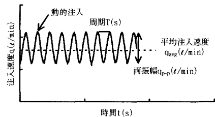
図2 動的注入の注入速度の波形例
