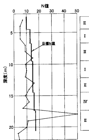
図-4. 原地盤のN値
