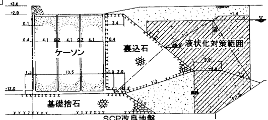
図-3. 施工断面図
