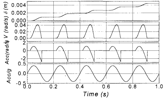
図5 時刻歴図
