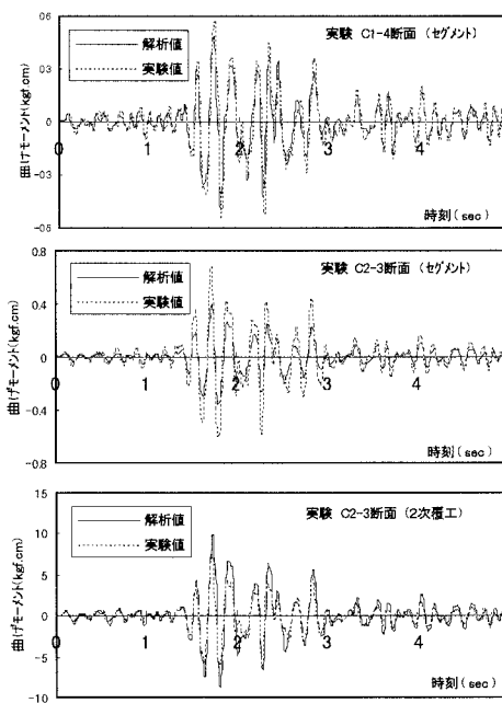
図6：三次元FEMをもとにした断面力の時刻歴
