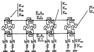
図 3. トンネルの解析モデル
